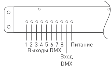
Рис. 4. Индикаторы дистрибьютора.
